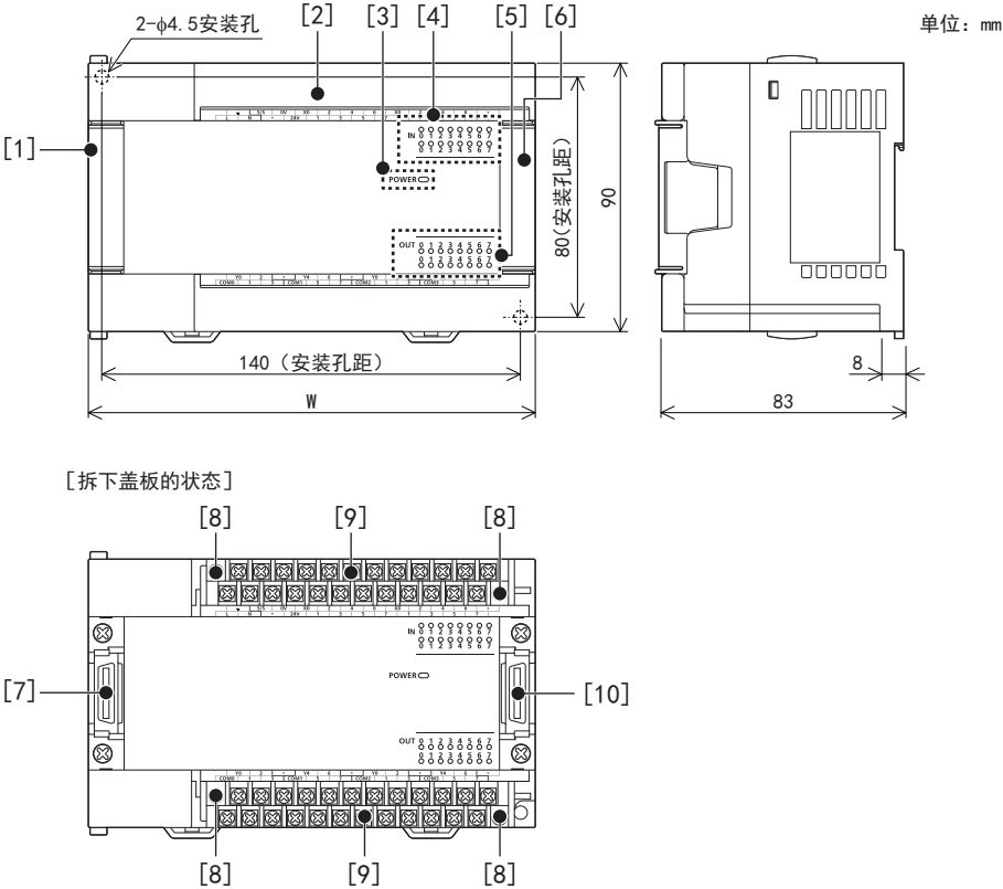
外形尺寸
