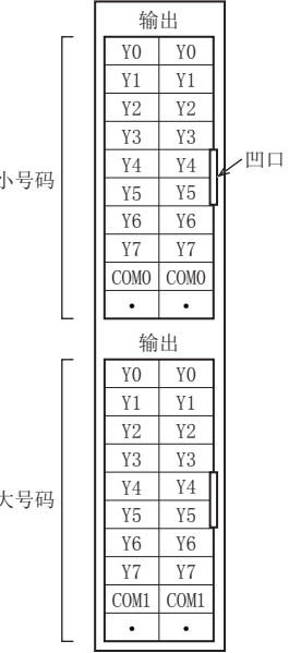
FX5-C32EYT/DSS
