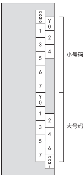
FX5-16EYR/ES FX5-16EYT/ES
