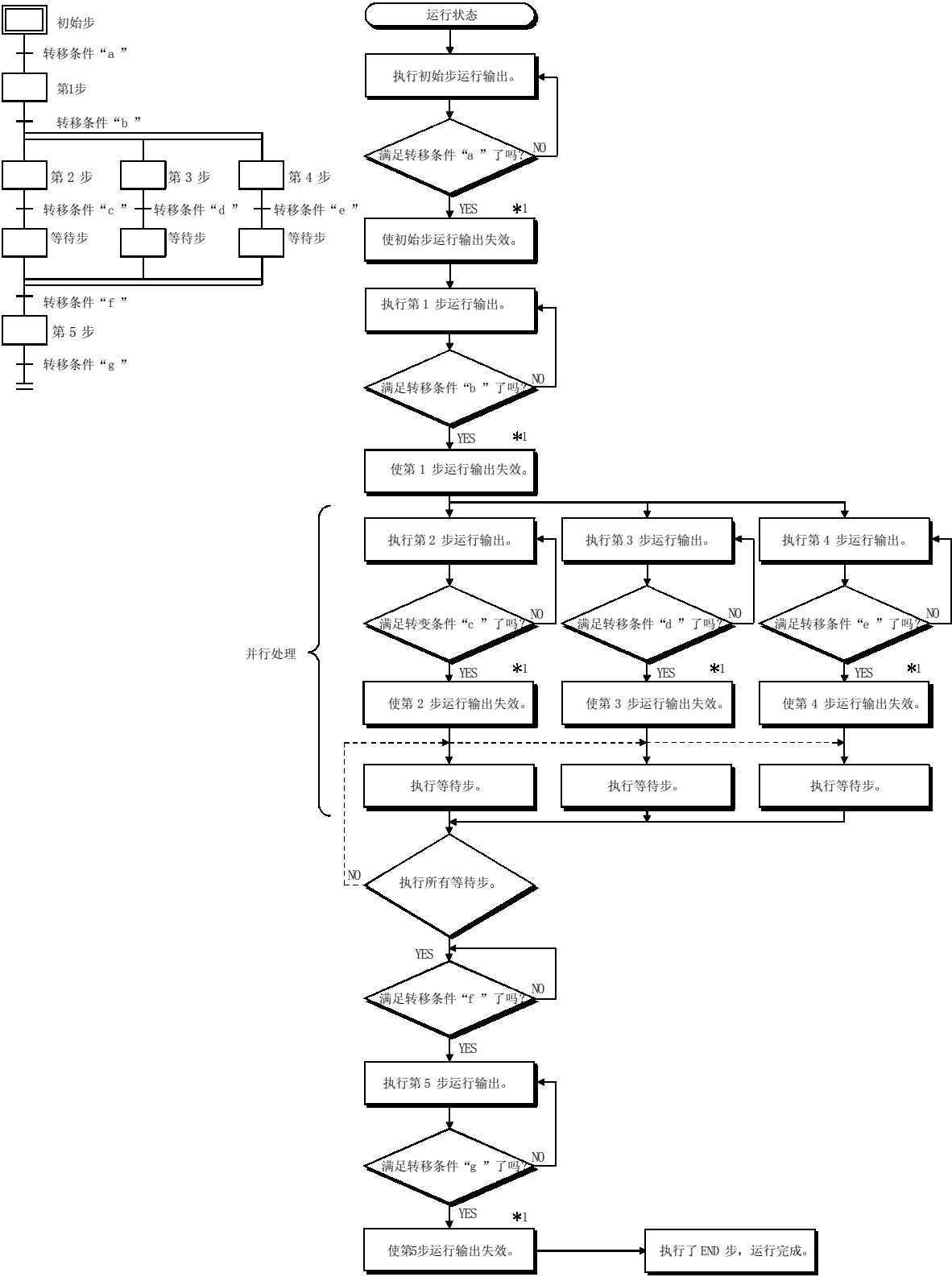
(6) 并行转移运行流程图
