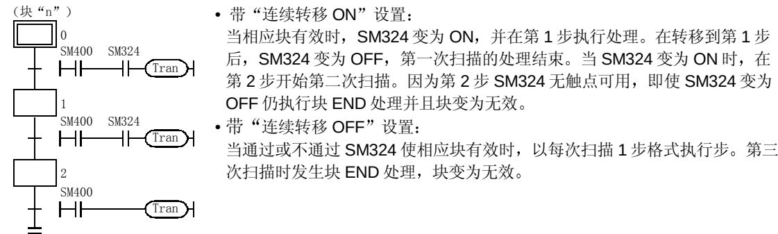
例 2: 通过样例程序处理（带“连续转移 OFF”标志）
