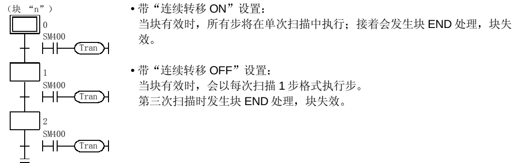
例 1: 样例程序和相应的处理（带“连续转移 OFF”标志）
